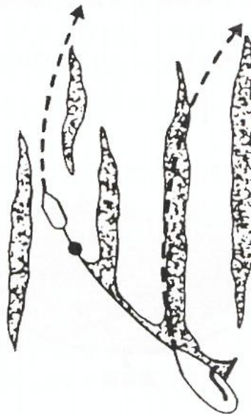
图 5-8 单船收油系统另加一船拖曳围油栏，以增加围油率
